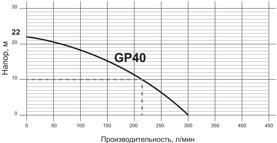
Рис. 24 График зависимости производительности мотопомпы от высоты подъема
