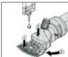
Рис. 4. Отверстия для смазки маслом.
