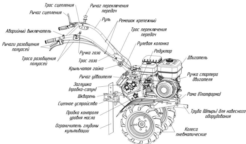
Рис.1 Мотоблок общий вид (вид справа)
