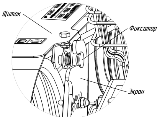
Рис.4 Схема крепления щитка со стороны ведомого шкива
