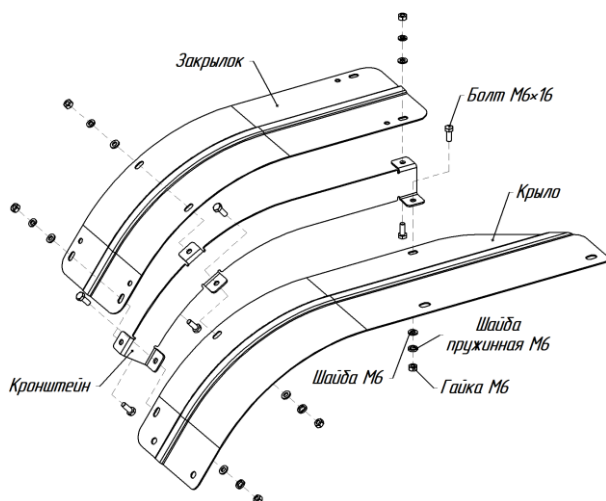
Рис.11 Схема крепления закрылков на мотоблоках МБ23 МА-ZS (GB390) и МБ23 МА-ZS (GB390) М
