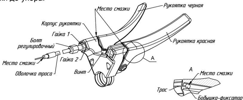
Рис.14. Заделка тросов разобщения в рукоятке
