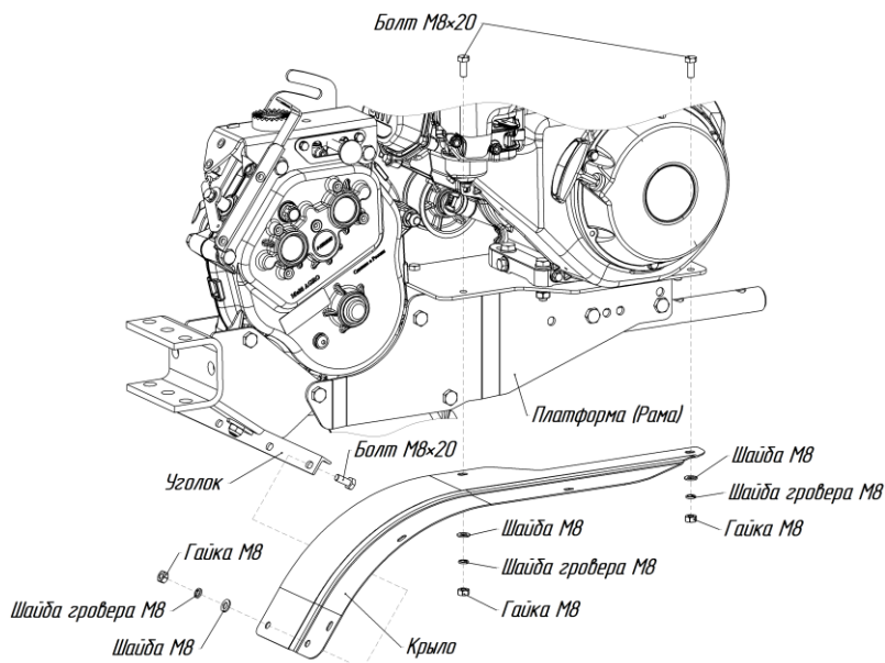
Рис.13 Установка крыльев на мотоблоки МБ23 МА-ZS (GB390) и МБ23 МА-ZS (GB390) М
