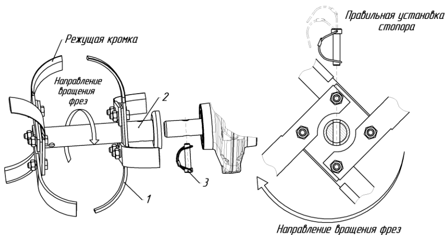
Рис.19. Схема установки 4-х фрез-культиваторов 1-нож; 2-ступица; 3-стопор
