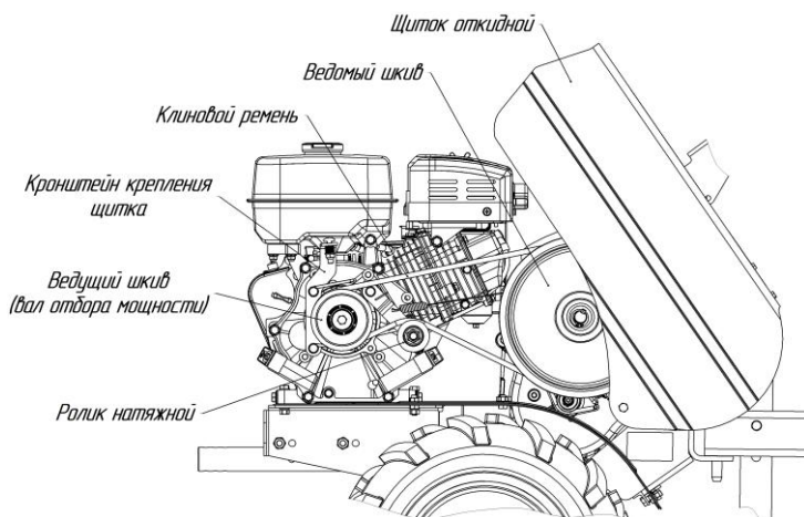
Рис.2 Мотоблок вид слева (щиток поднят)
