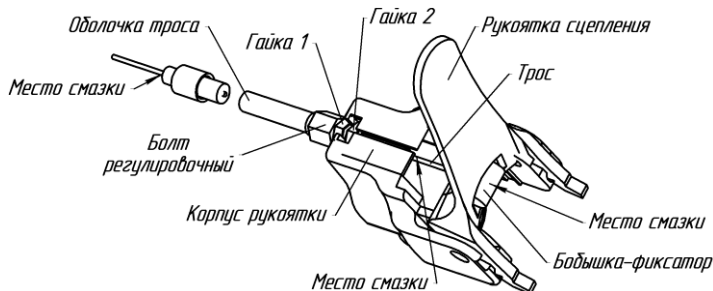
Рис.7 Заделка троса в рукоятке сцепления
