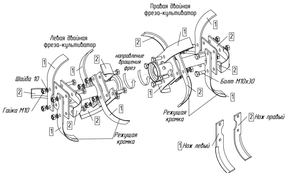
Рис.17. Схема сборки двойных фрез-культиваторов
