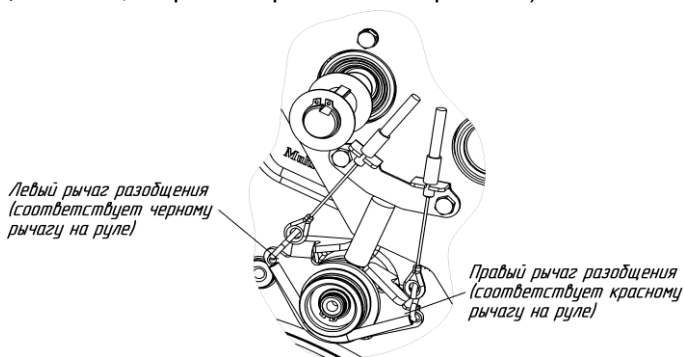
Рис.16 Соответствие рычагов разобщения на редукторе и на руле мотоблока при присоединении тросов разобщения
