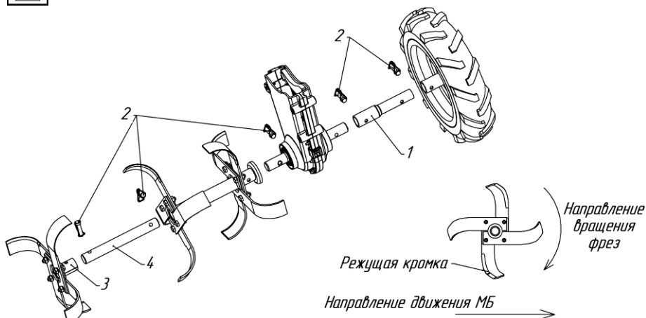
Рис.18. Схема установки 6 фрез-культиваторов или колес 1-удлиннитель полуосей; 2-стопор; 3-фрезы; 4-валик
