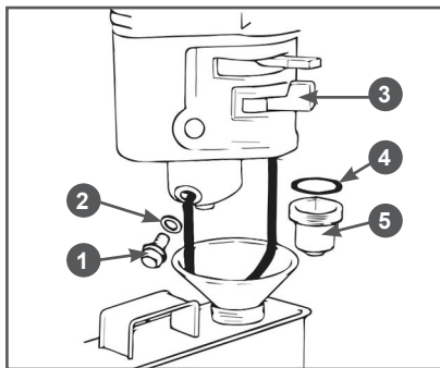
Рис. 19 Обслуживание фильтра-отстойника
