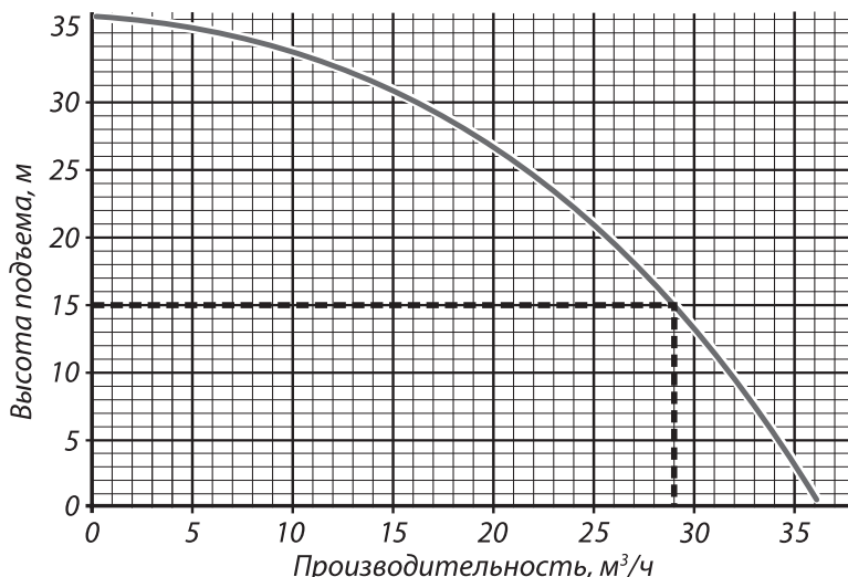
Рис. 22 График зависимости производительности мотопомпы от высоты подъёма
