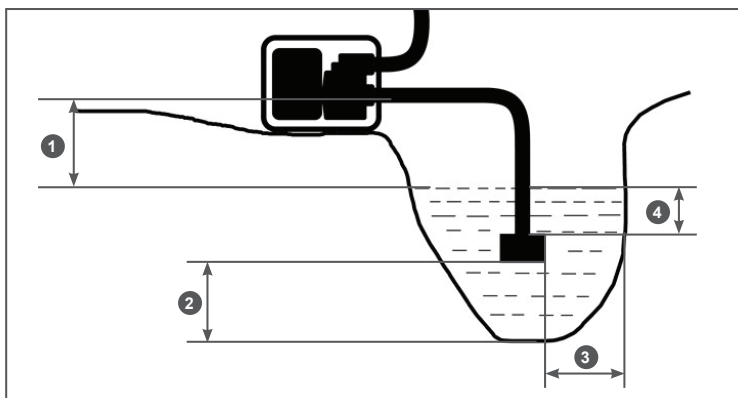
Рис. 9 Расположение мотопомпы и всасывающего фильтра
