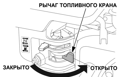
Рис. 16 Рычаг топливного крана
