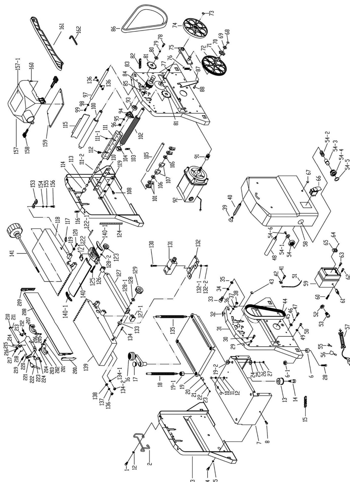
Рисунок 14. Взрыв-схема для модели BELMASH JT-2 204/210
