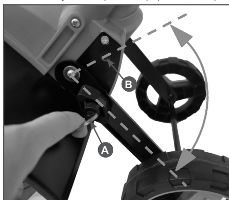
Рис. 3 Изменение положений колес
