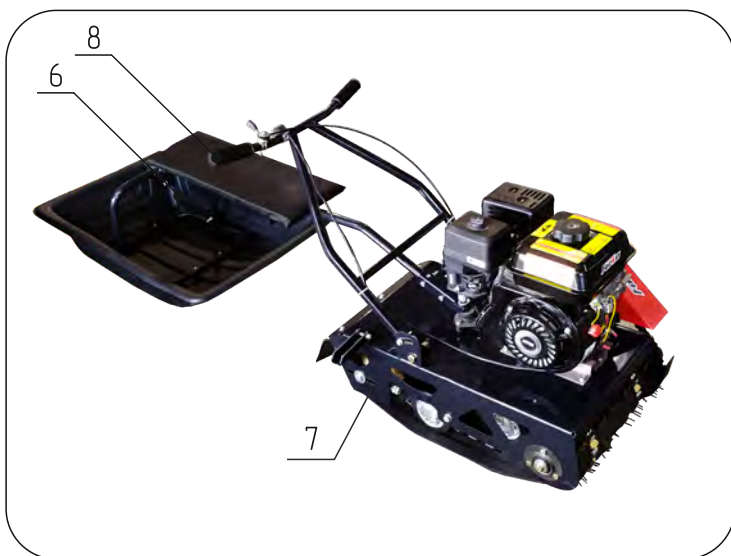
Рис. 10. Мотобуксировщик МБС 4С. Вид справа.
