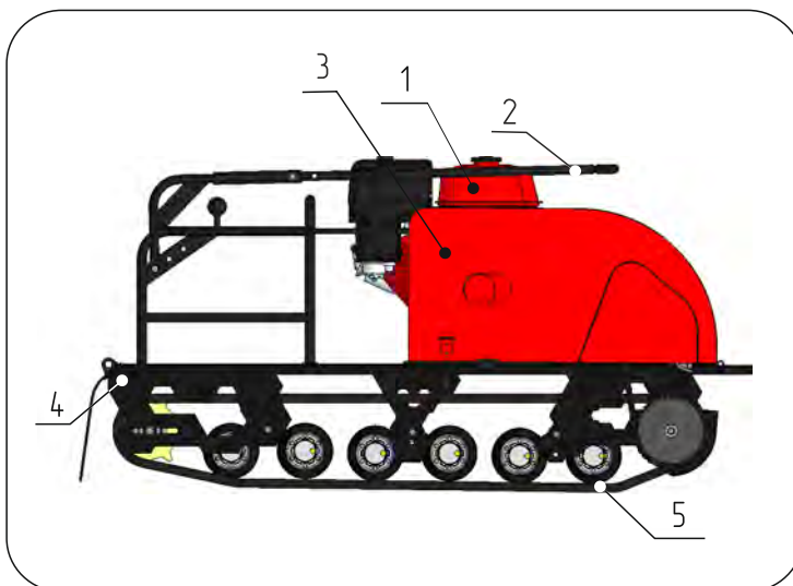
Рис. 11. Мотобуксировщик МБС 5. Вид слева.
