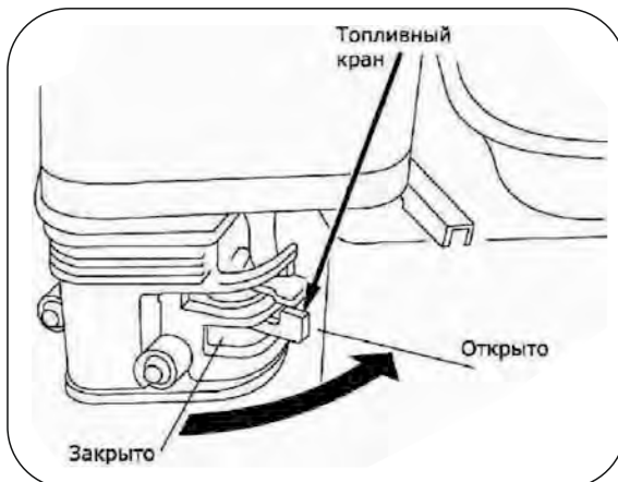
Рис. 14. Управление топливным краном и заслонкой обогатителя.
