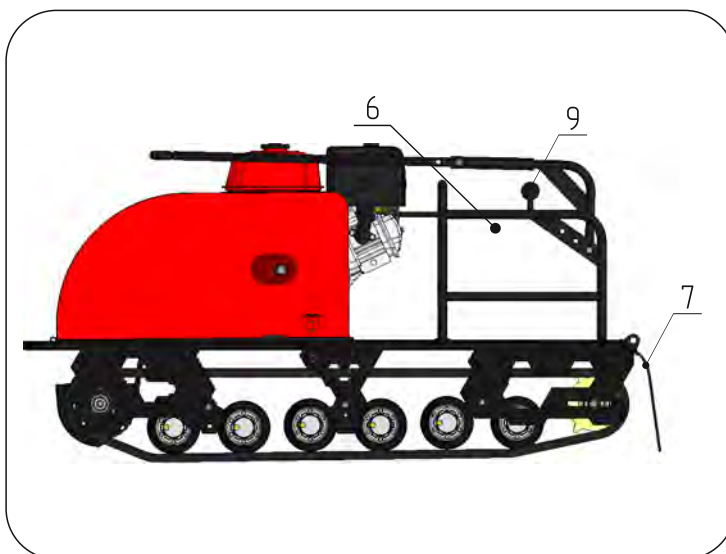
Рис. 12. Мотобуксировщик МБС 5. Вид справа.
