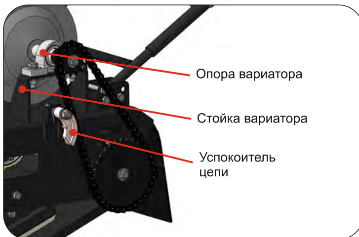
Рис. 16. Регулировка натяжки цепи МБС 3С.
