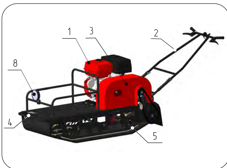
Рис. 7. Мотобуксировщик МБС 3С. Вид слева.
