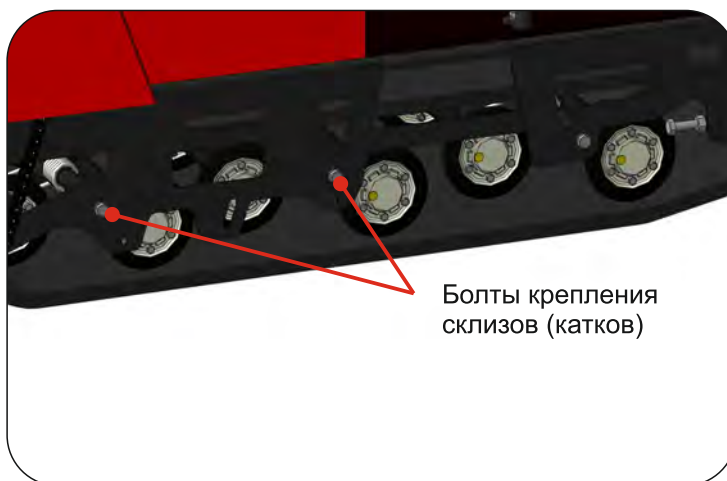
Рис. 19. Регулировка угла «атаки» МБС 3, МБС 5.
