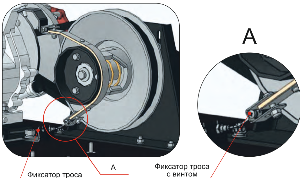
Рис. 23. Тормозная система (опционно).
