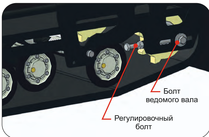
Рис. 17. Регулировка натяжки гусеницы.
