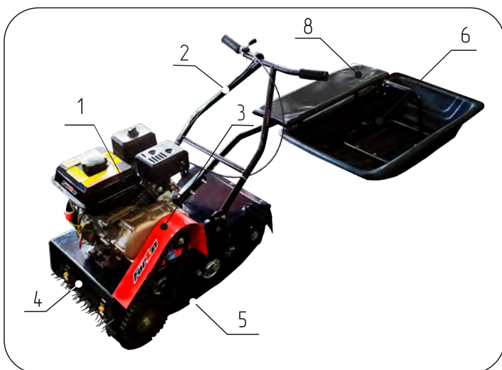
Рис. 9. Мотобуксировщик МБС 4С. Вид слева.
