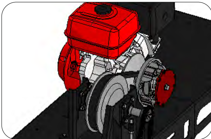
Рис. 15. Регулировка натяжки цепи МБС 2, МБС 3.
