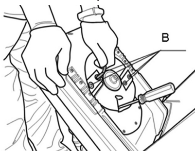
Рис. 9. Снятие ножей
