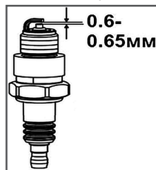
Рис.15 Свеча зажигания
