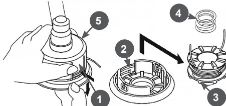
Рис. 17 Разборка триммерной головки
