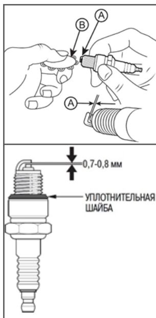
Рис. 23 Зазор между электродами свечи зажигания
